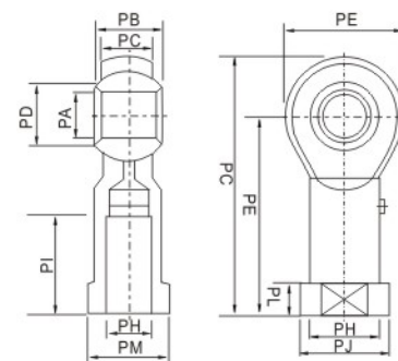
M-PHS 型鱼眼接头
